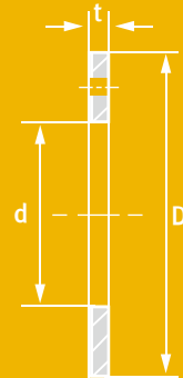
TFA/P Anlaufscheiben
