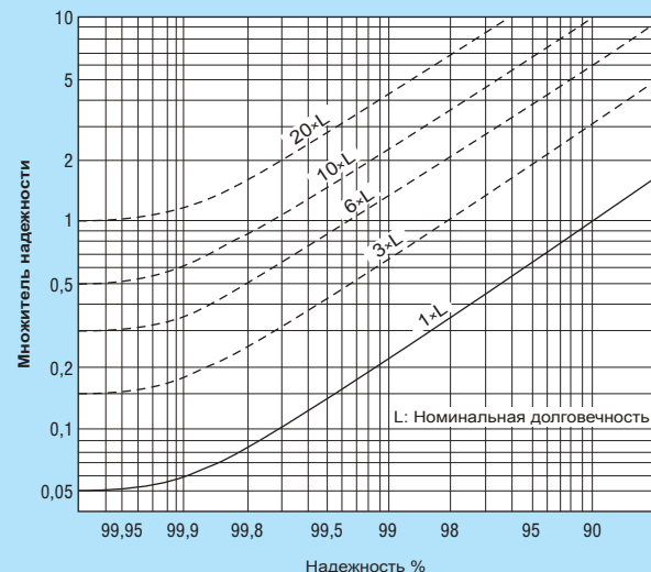
Рис 3.6 График надежности
