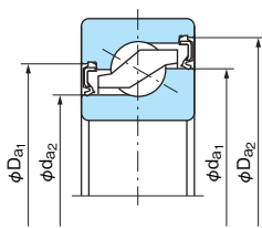
С контактными уплотнениями (2LR)
