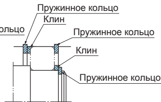
(с) Пружинное кольцо и прокладка с выемкой
